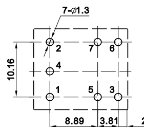
安装孔位图 (底视图)
