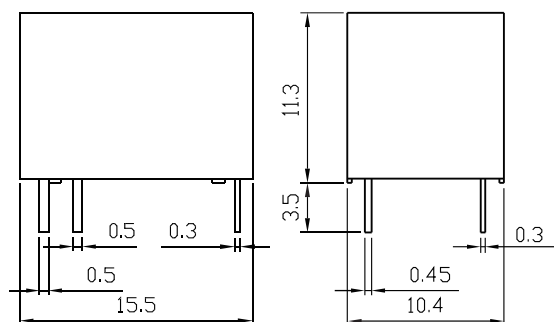
外形尺寸 Outline Dimensions
