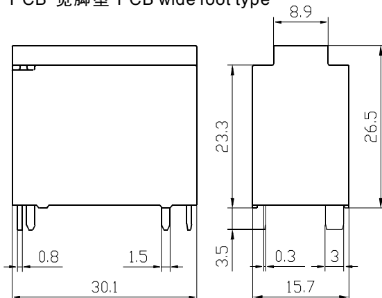
PCB-宽脚型 PCB wide foot type
